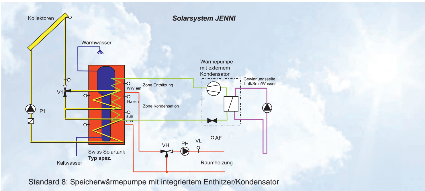
Speicher Swiss Solartank mit integriertem Boiler, Solar- und Wärmepumpen-Tauscher
