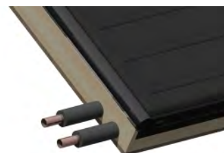
Anschlüsse durch den Kollektorrahmen: z.B. bei Fassadeneinbau (bei Indach- montage mit Eindeckrahmen nicht möglich).
