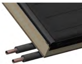
Anschlüsse in Lattenhöhe: Leitungen können unter den Dachziegeln verlegt werden (nur bei VarioSol E).
